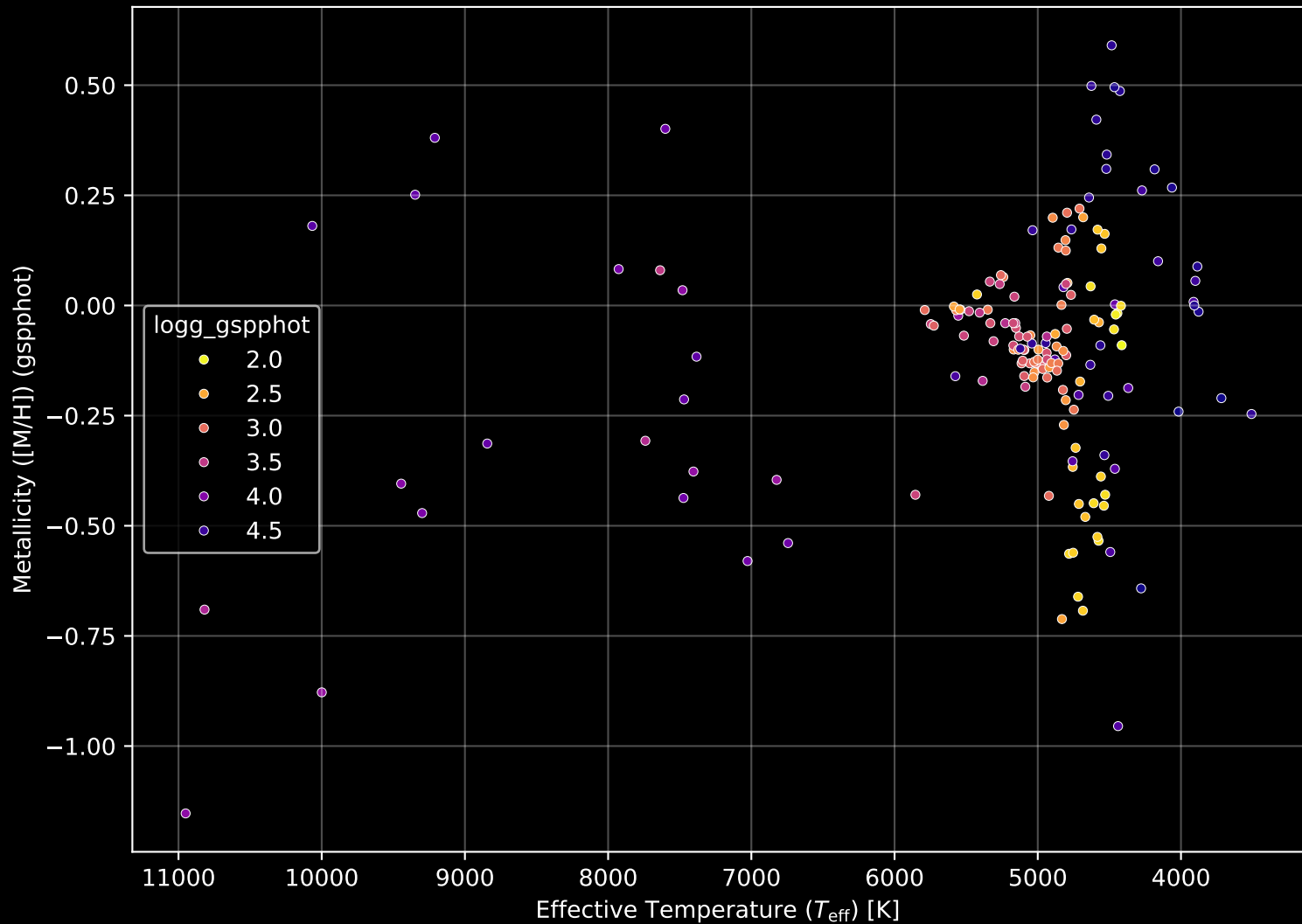
APOGEE DR17 Field: [165+18] Stellar Population Parameters (n= 167)
